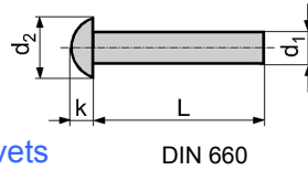
DIN 660
