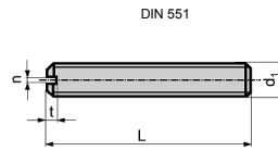
DIN 551
