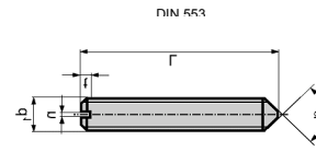
DIN 553
