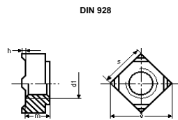
DIN 928
