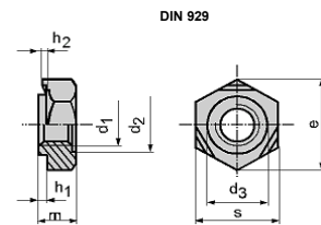
DIN 929
