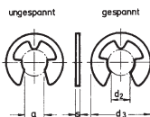
DIN 6799
